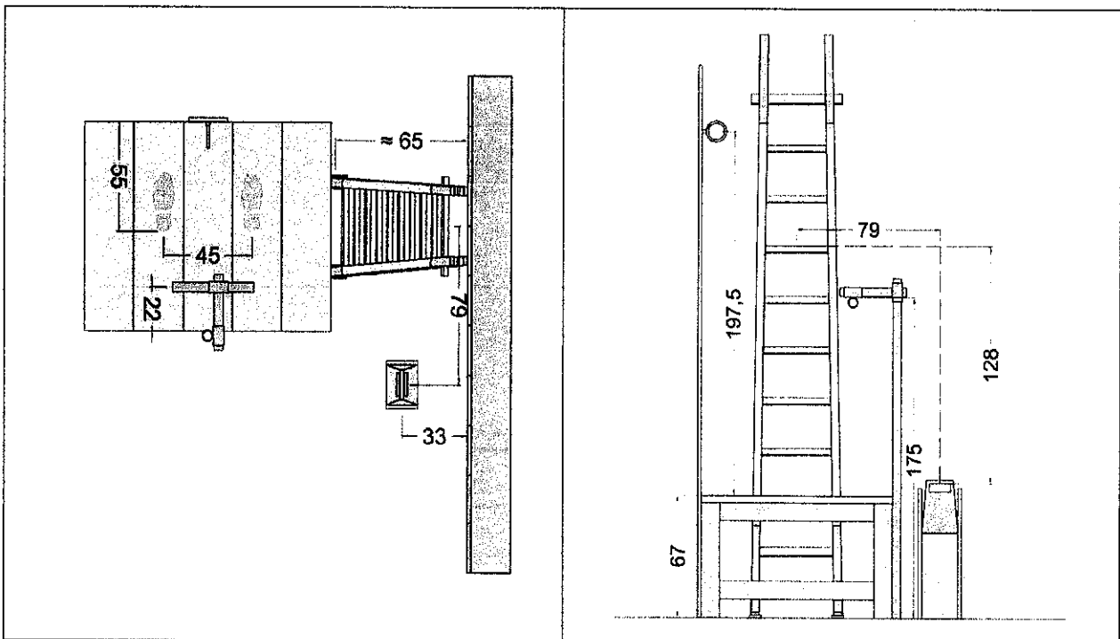
figura 9: Pianta e prospetto della postazione
